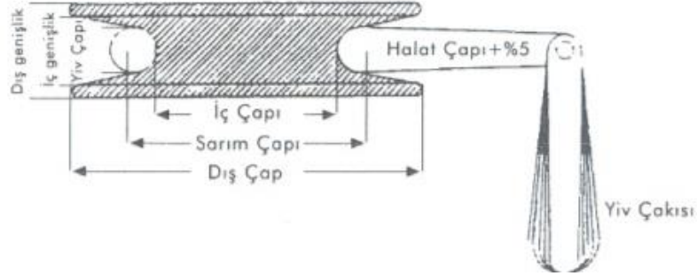
Şekil-6. Bazı makara boyutları ve yiv çakısı kullanımı
