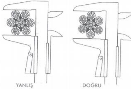
Şekil-3. Halat Çap ölçüm yöntemi
