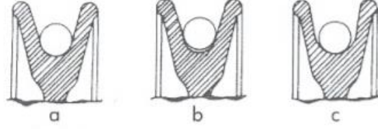
Şekil-5. Makara yiv kesitleri a)Yeni halat-yeni yiv, b)Yeni halat-aşınmış yiv, c)Aşınmış halat-aşınmış yiv
