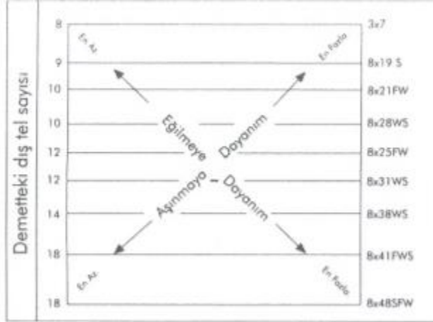
Şekil -4. Halat Kompozisyonuna göre esneklik ve aşınma direnci eğilimi
