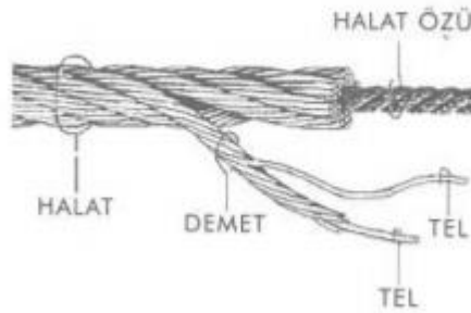
Şekil-1 Halatı meydana getiren elemanlar
