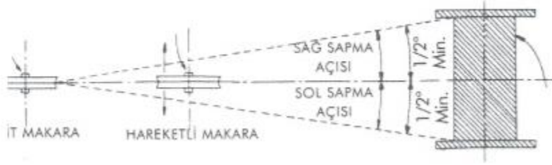
Şekil -7. Halat kullanımında sapma açısı
